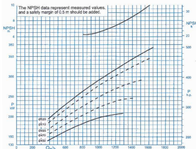
منحنی عملکرد
