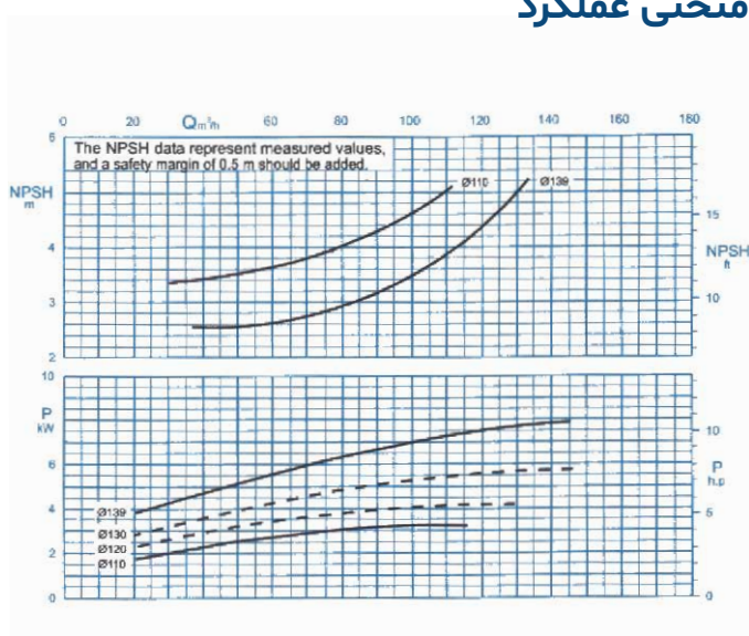
منحنی عملکرد
