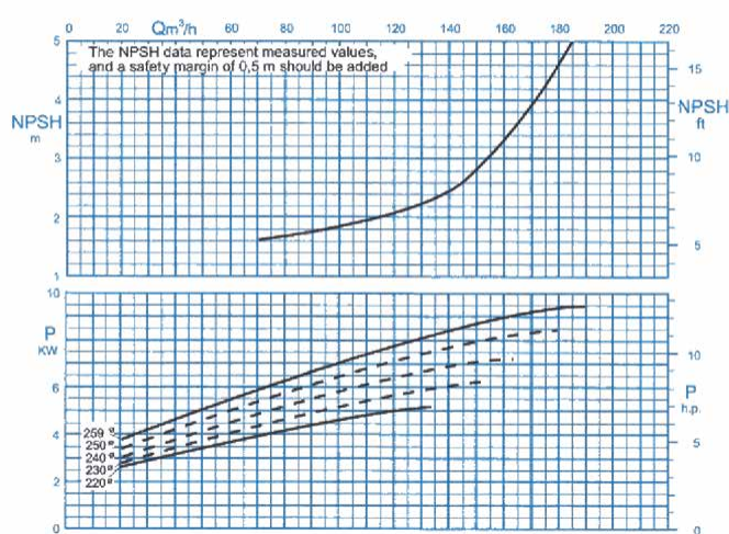
منحنی عملکرد
