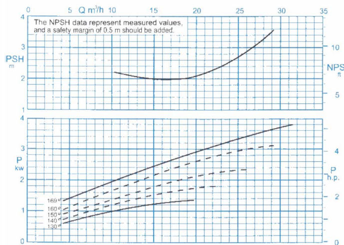
منحنی عملکرد
