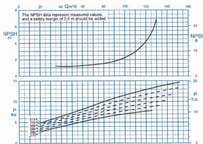
منحنی عملکرد
